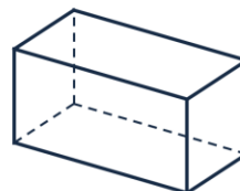
Paralelipipedul dreptunghic
